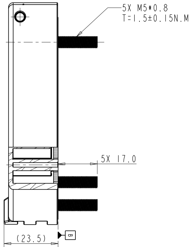
截面 A-A
